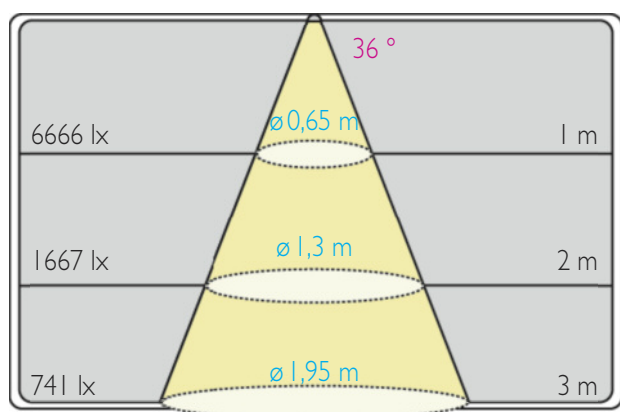
ALTIS 2700 K LENTILLE 36°
