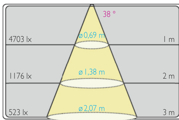
ALTIS 4000 K REFLECTEUR 38°
